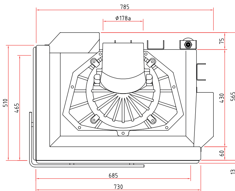
Draufsicht M 1:10
