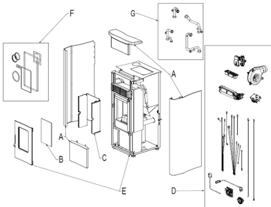
Rys. 1 - Rysunek rozstrzelony
